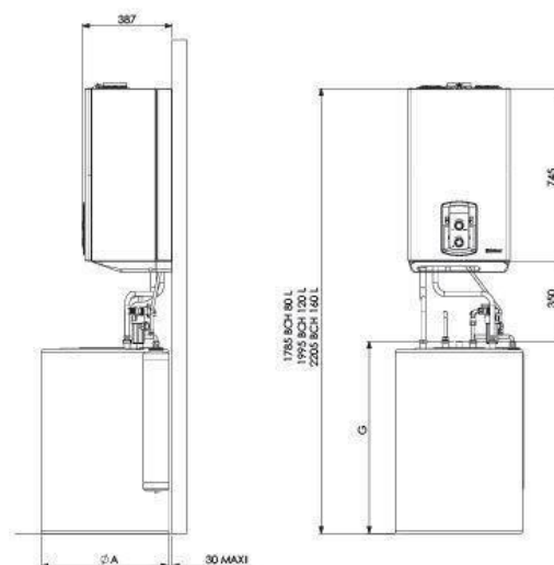
Ballon BCH placé sous la chaudière. Référence : 3318335
