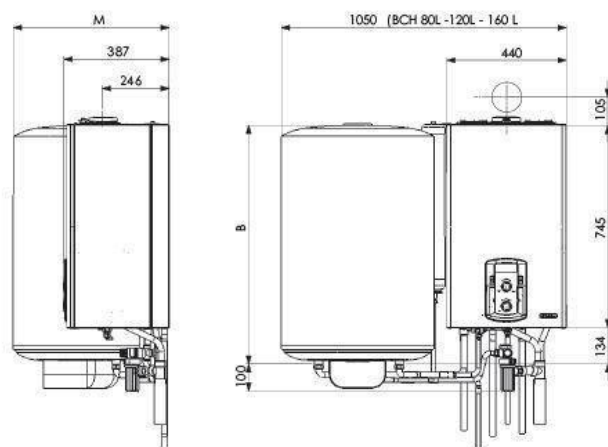
Ballon BCH placé au mur à gauche de la chaudière. Référence : 3318630
